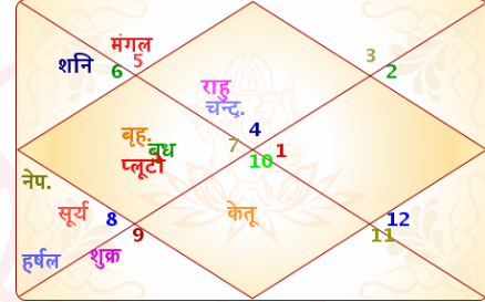
चन्द्र कुण्डली
