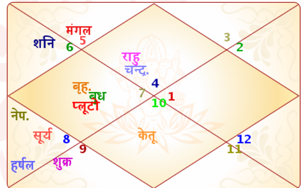
चन्द्र कुण्डली
